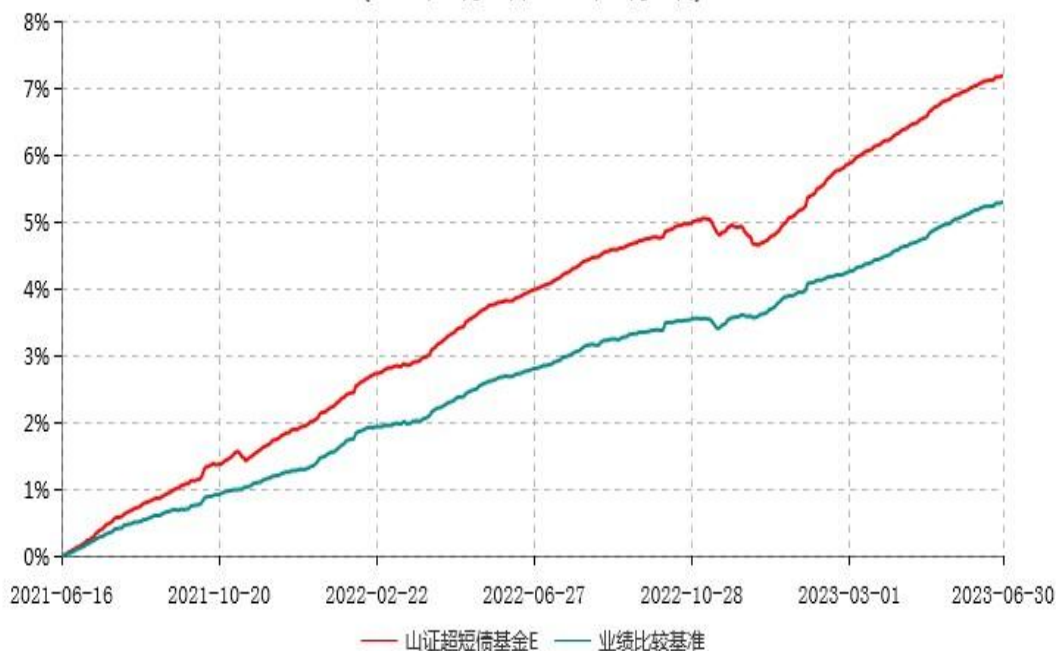
山证超短债基金E累计净值增长率与业绩比较基准收益率历史走势对比图 (2021年06月16日-2023年06月30日)
